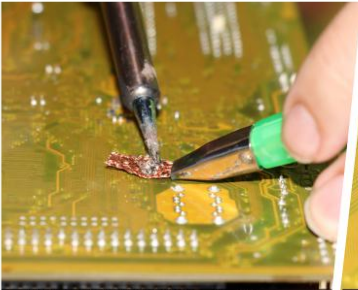
然后用电烙铁轻压加热
