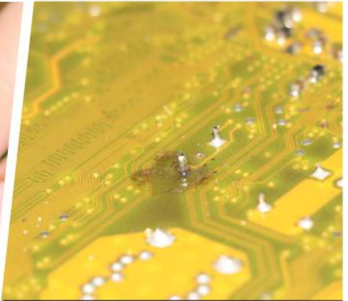
焊锡融化后即被吸锡线吸取
