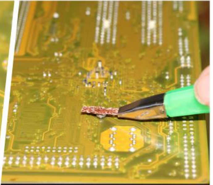
将适当长度的吸锡线置于被清理的焊点上
