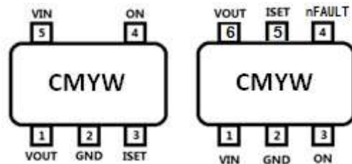
SOT23-5
